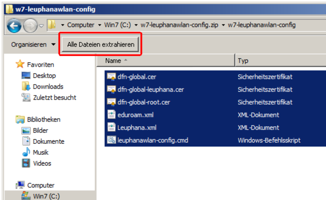
Abbildung 1: Konfigurationspaket entpacken
