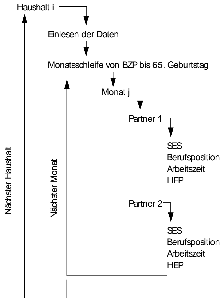
Abb. 3: AVID-PRO: Zum Ablauf des Simulationsprozesses
