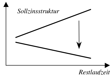
Abb. 2: Sollzinsstruktur bei optimalem Wachstum
