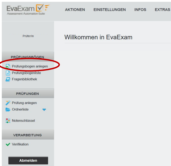
Abb. 1: Prüfungsbogen anlegen
